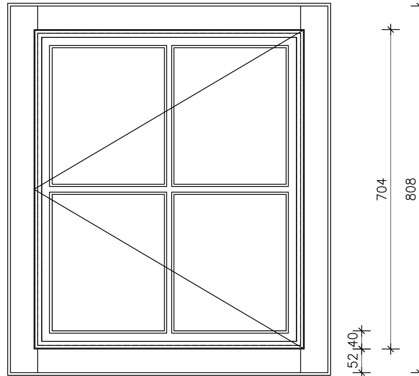
Aussenflügel, Aussenansicht 1:5
